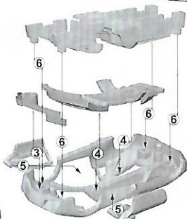
车门拼装图
